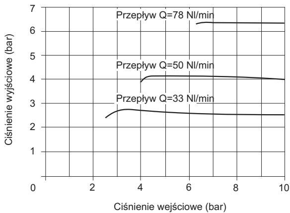
Charakterystyki regulacji
