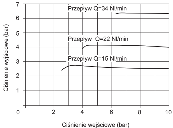
Charakterystyki regulacji
