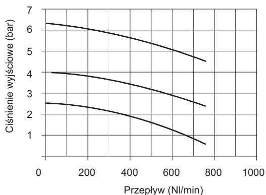
Charakterystyki regulacji
